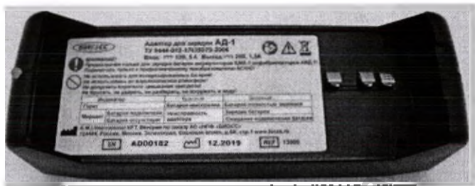
а) адаптер для зарядки батареи аккумуляторов АД-1.
