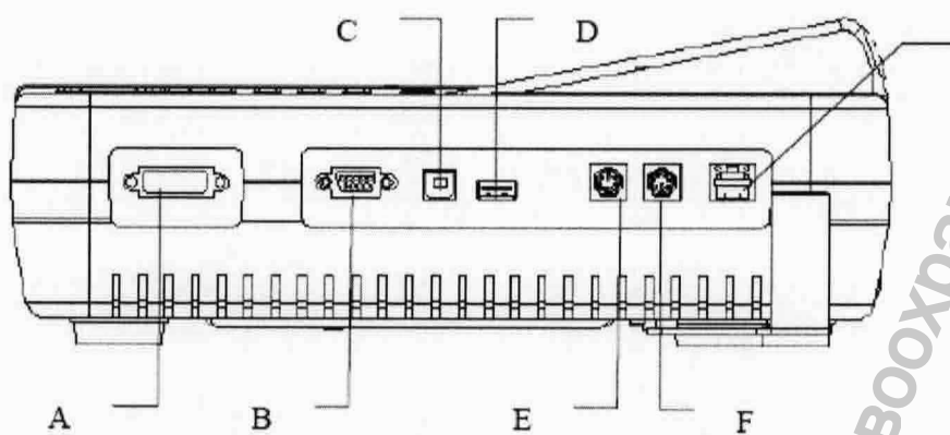
Рис.6-6. Правая панель кардиографа ЭКГ-10-12.
