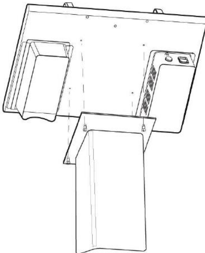
Рис. 4 Сборка стола
