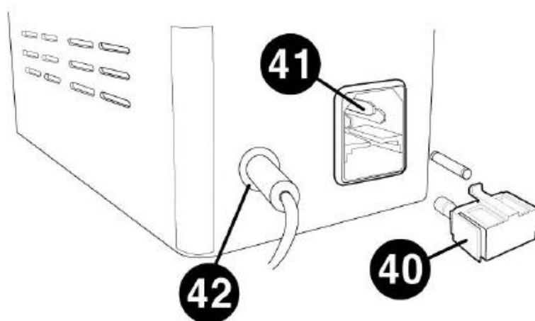
Рис. 8 Замена предохранителей
