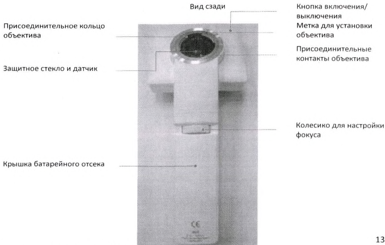
Вид сзади
