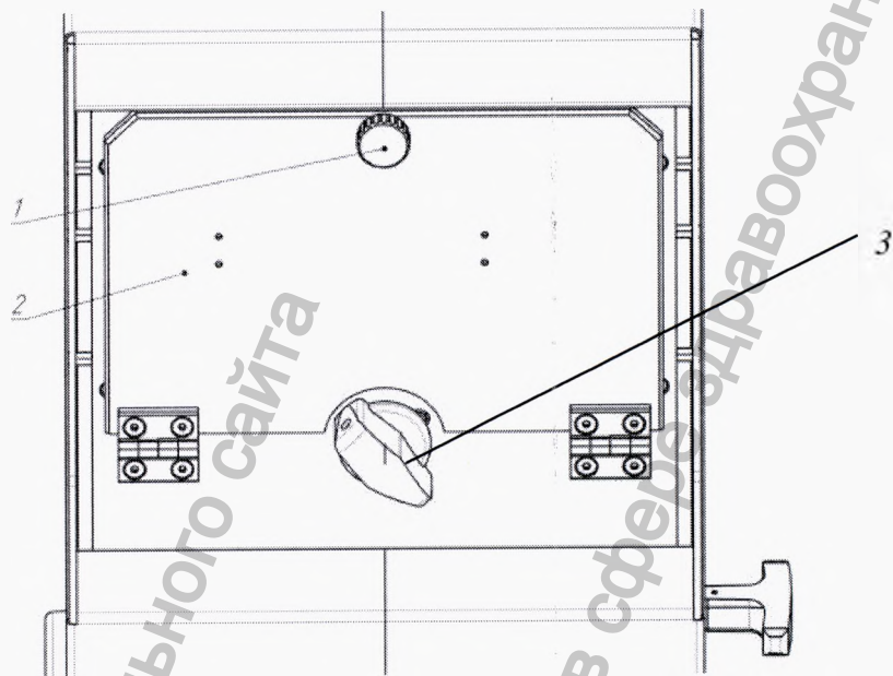
1 – винт, 2 – крышка 3 – рукоятка переключения ламп Рисунок 27 – Внешний вид
