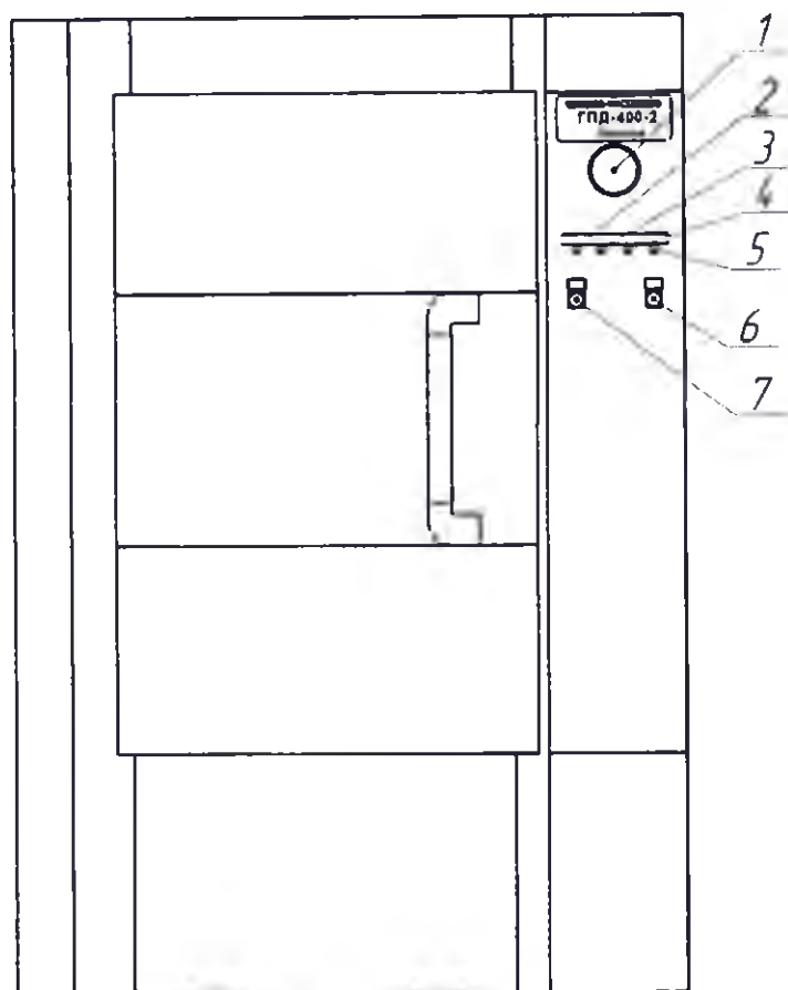
Рисунок 2 - Стерилизатор паровой с автоматическим управлением ГПД-400-2-«ТЗМОИ». Вид со стороны стерильной зоны (схематичный эскиз)
