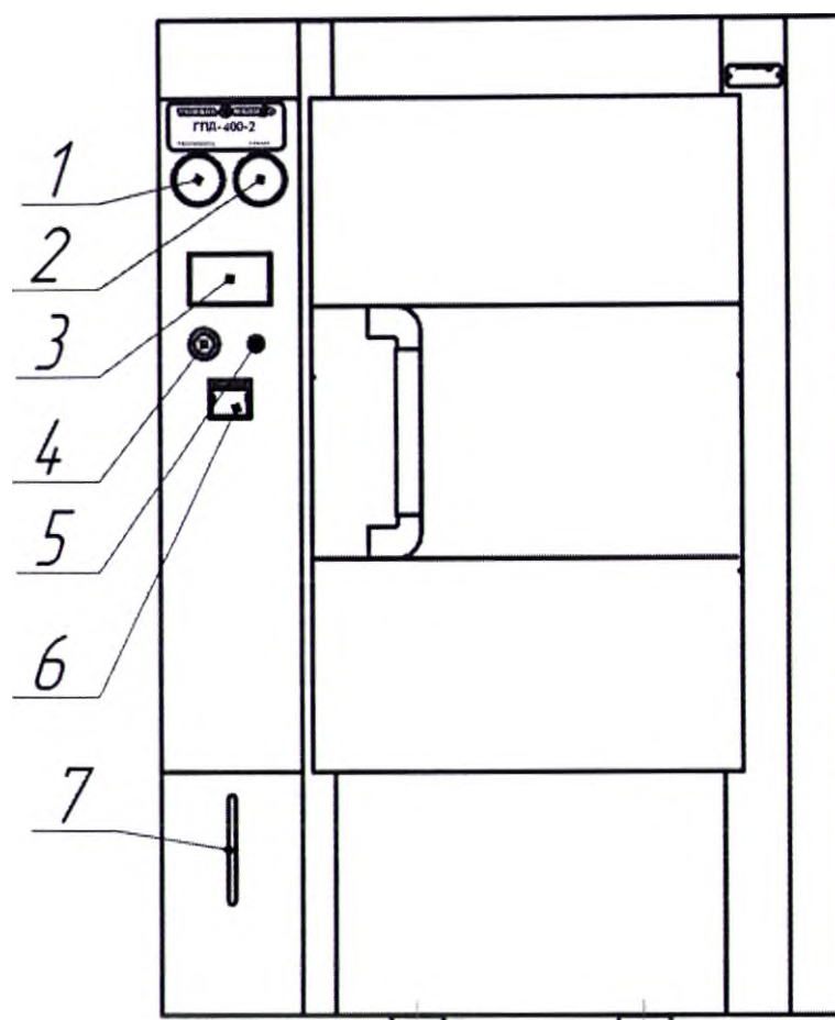
Рисунок 1 - Стерилизатор паровой с автоматическим управлением
