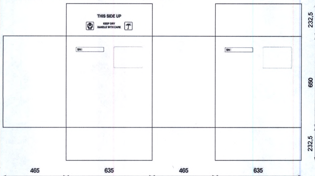
[Изображение 36] Транспортная коробка URK-800A
