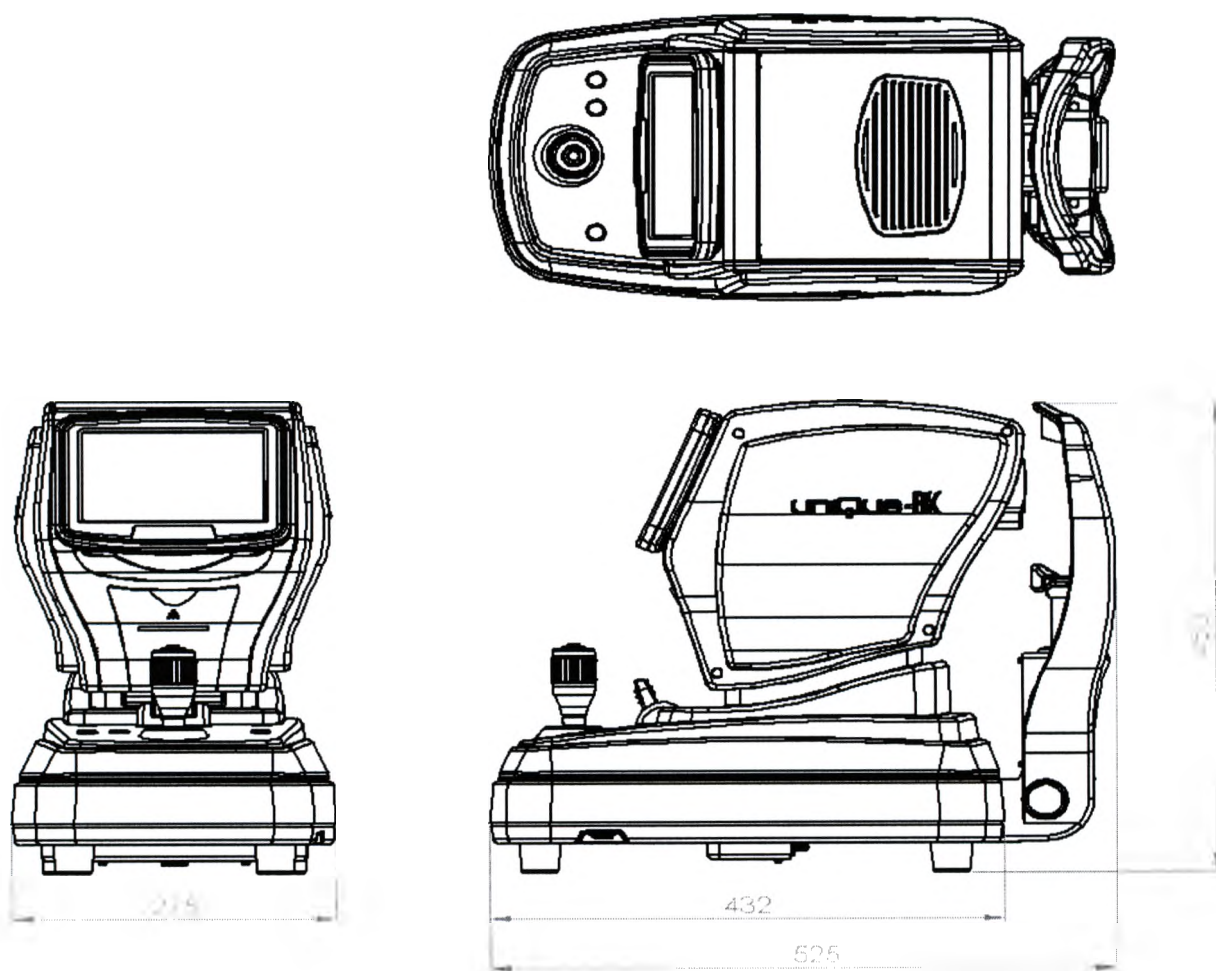
Рисунок 20 – Габаритные размеры авторефрактокератометра
