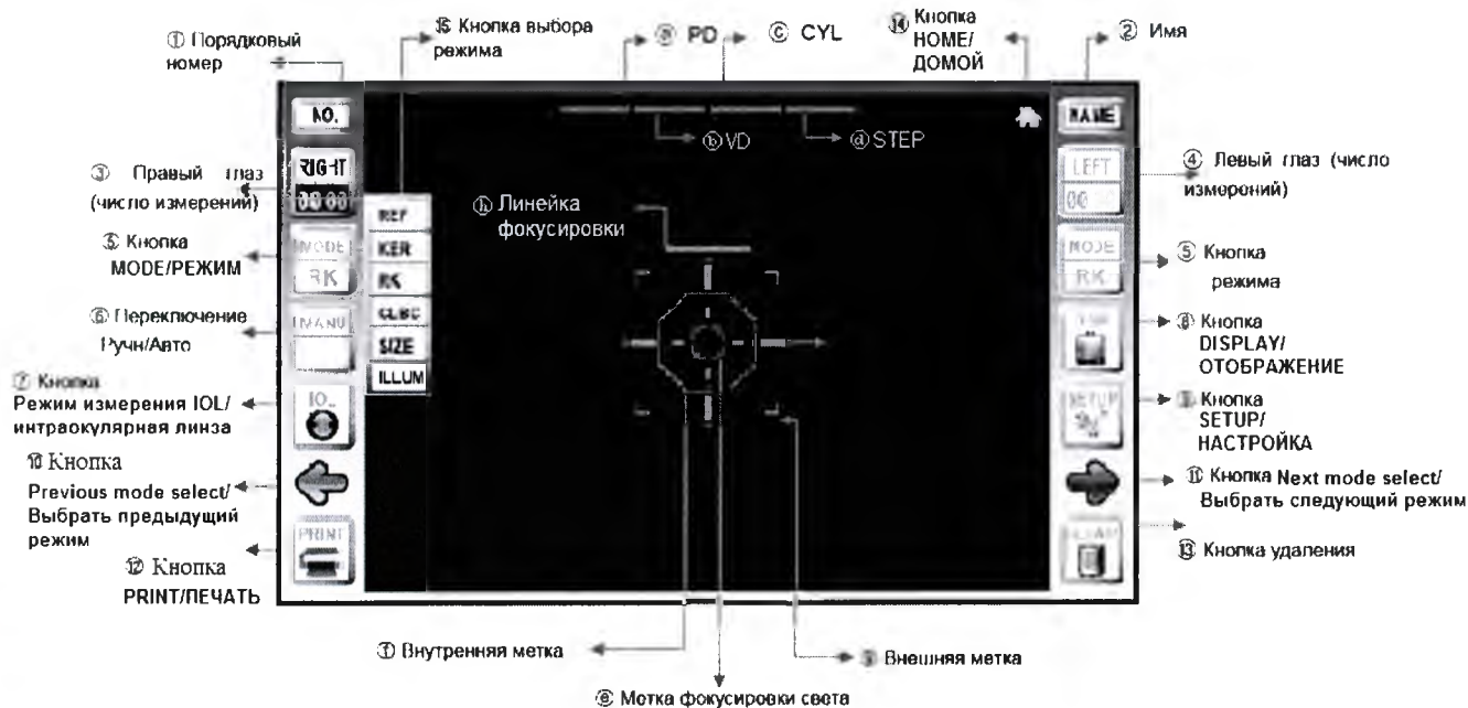
Рисунок 21 – Пользовательский интерфейс
