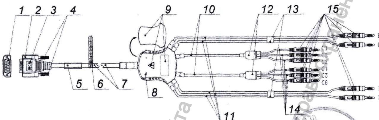
Рисунок 2.1.5.1 – Конструкция кабеля ЭКГ с разъемами типа Vanapa (вид с обратной стороны).
