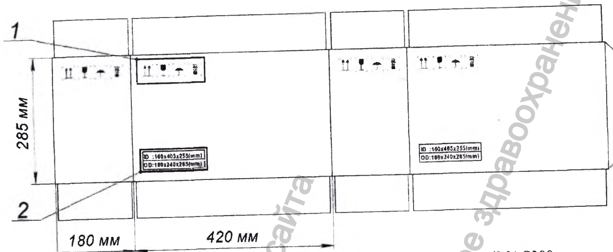
Рисунок I.7.2.1 – Макет транспортной тары варианта исполнения iMAC300 (1 – Символы условий транспортирования и хранения; 2 – Размеры транспортной тары, мм, \pm 5\% , ID – внутренние, OD – внешние, мм - мм).
