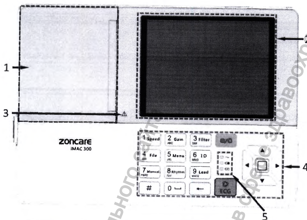
Рисунок 2.1.2.1 – Блок основной iMAC300 (вид сверху).
