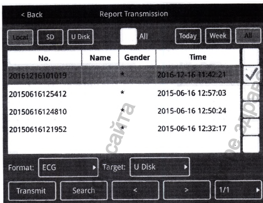
Рисунок 7.2 - Перемещение отчетов
