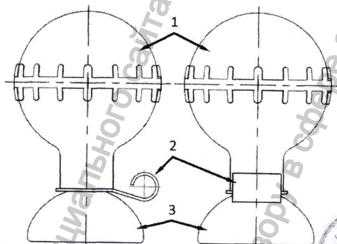
Рисунок 2.1.7.1 – Конструкция электрода грудного: 1 – груша, 2 – разъем электрода грудного, 3 – токосъемная поверхность
